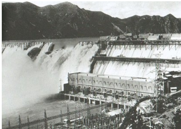
1937年 水力発電着工 1941年始動 1944年完成
