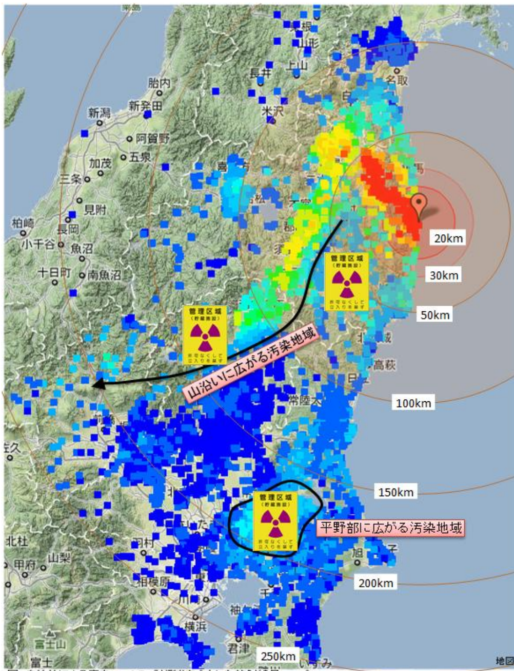
国・自治体による高さ1m・0.5m計測を中心とした放射線量マップ Radiation dose measured by MEXT and local governments at 1 or 0.5 meter height.
